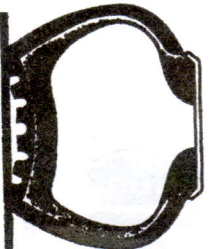
Podhuštěná pneumatika
